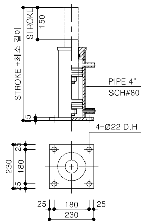
UP/DOWN HYDRAULIC SYLINDER 상세도
